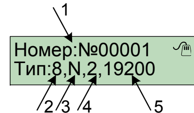
Рисунок 13. Экран конфигурации COM1
