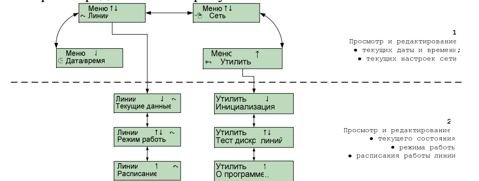
Рисунок 3. Структура меню контроллера «БиКуб-МТ02»
